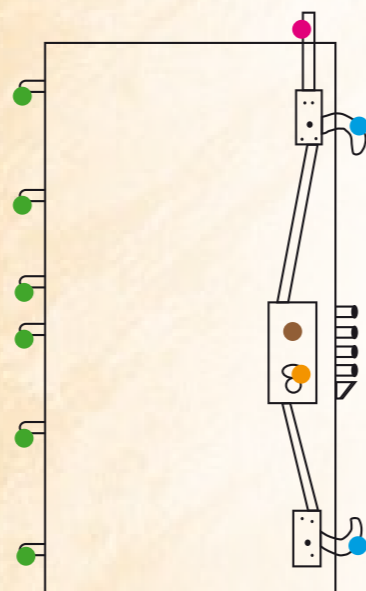
Figura 2: Limitatore di apertura laterale
